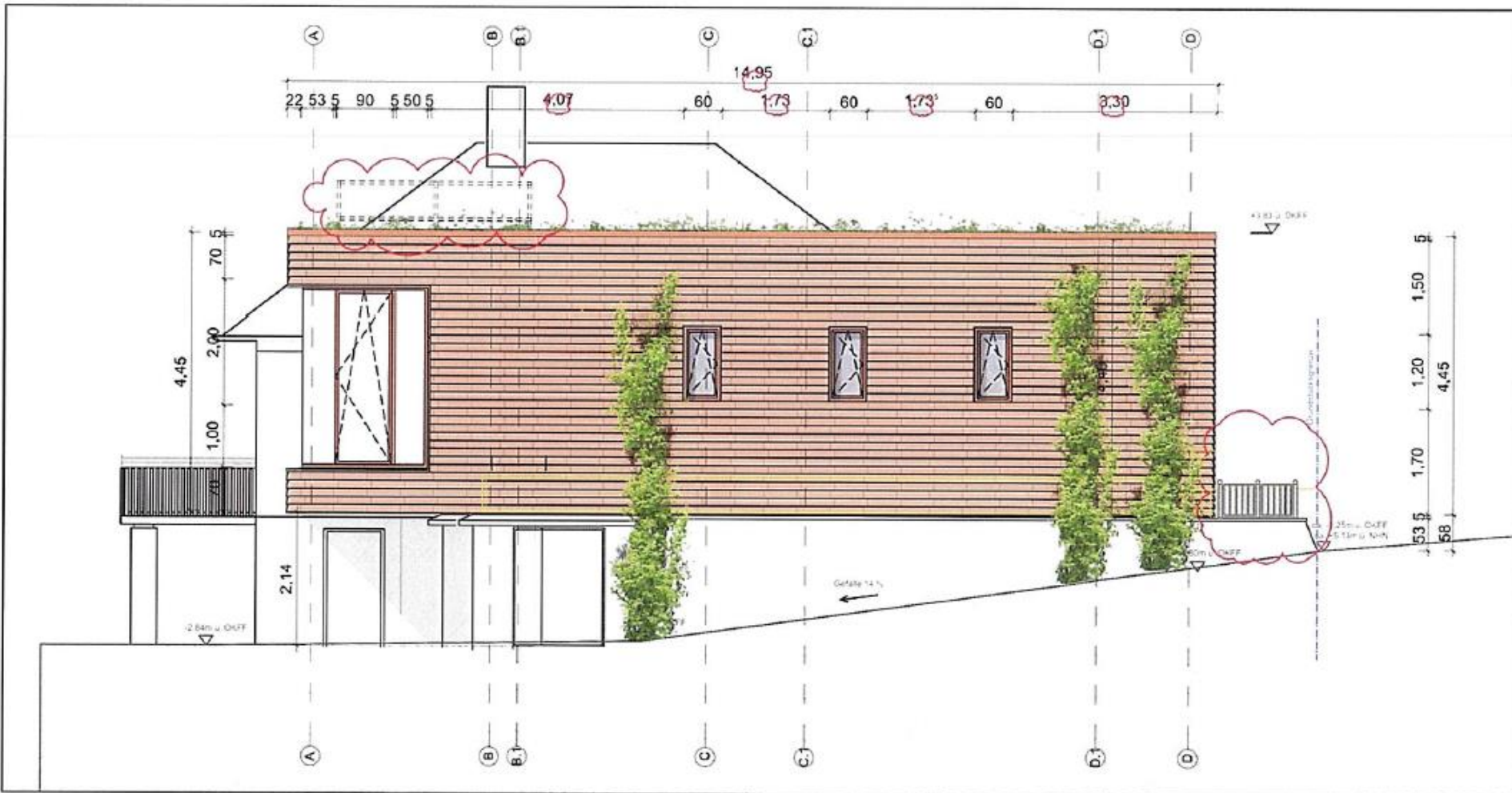
Ansicht Nord M 1:100
